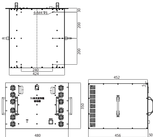
图 2 E82.C224K-I 机箱式压电控制器外形尺寸图
