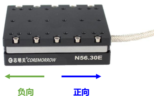
N56 系列直线压电马达位移台运动方向示意图
